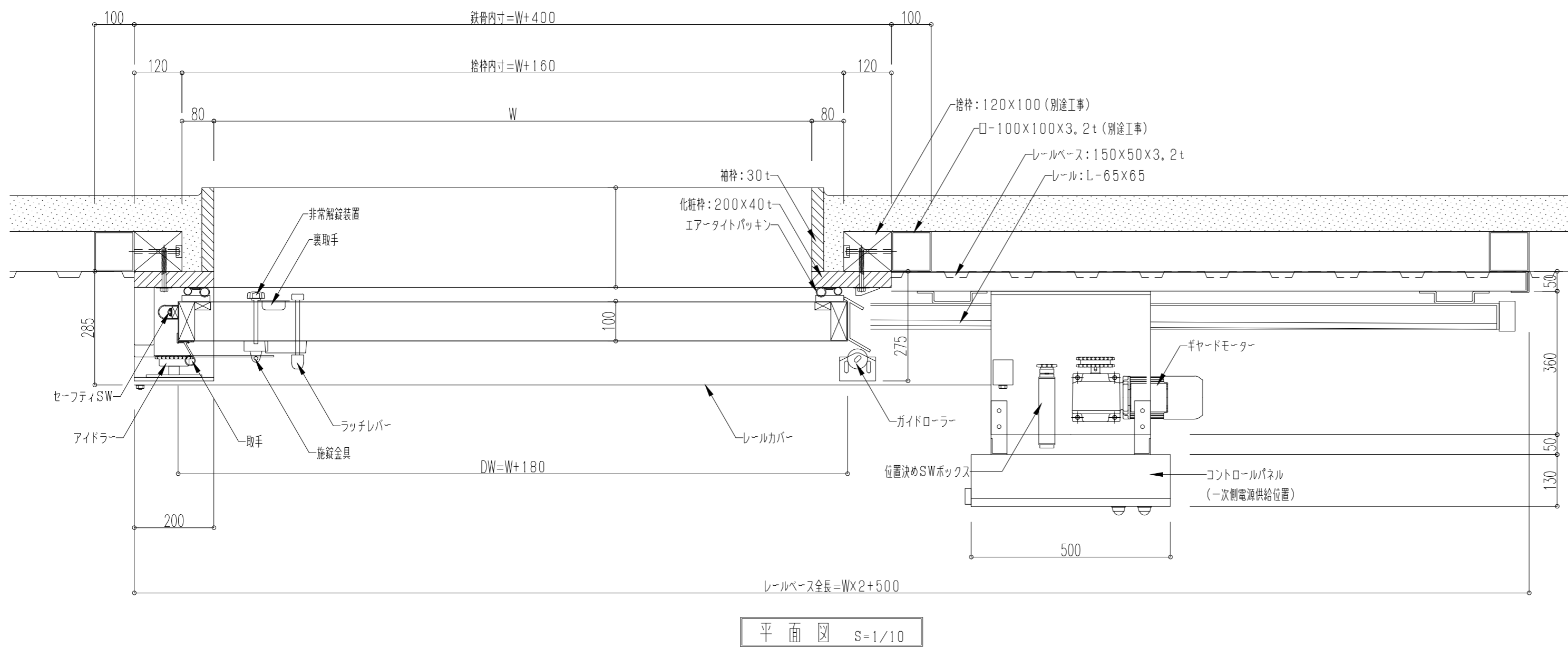
電動片引スライド扉(100t)
