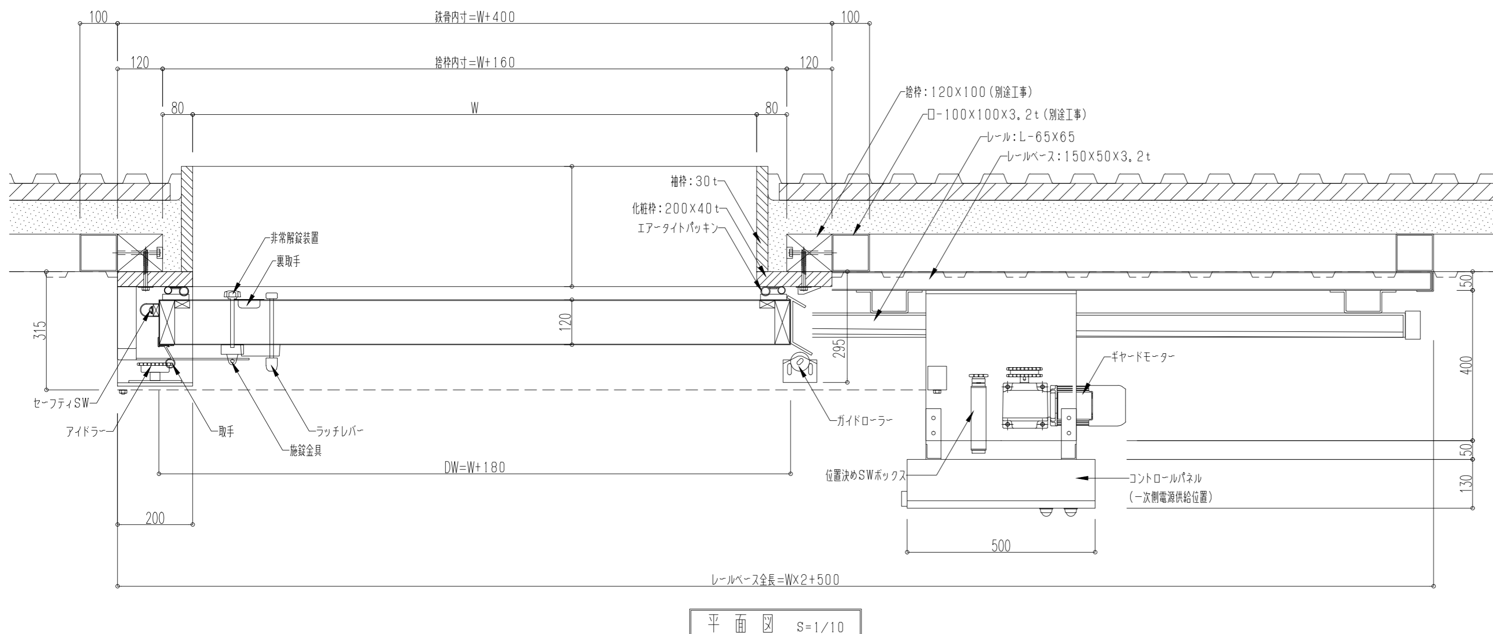
電動片引スライド扉(120t)
