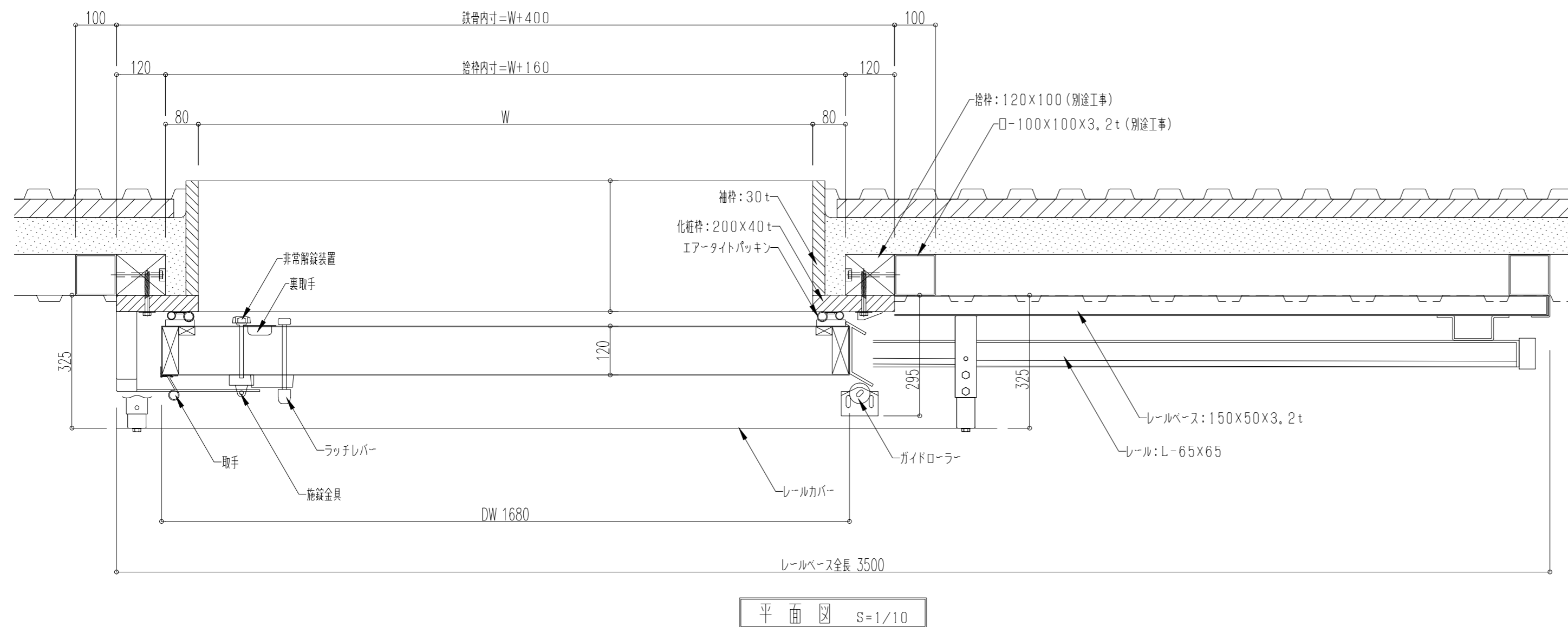
手動片引スライド扉(120t)
