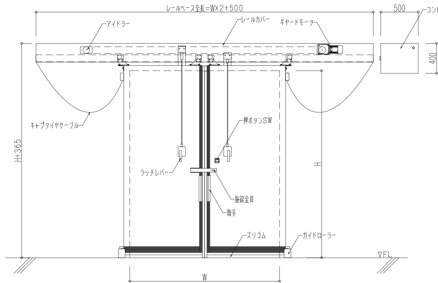
正面姿図 S=1/30
