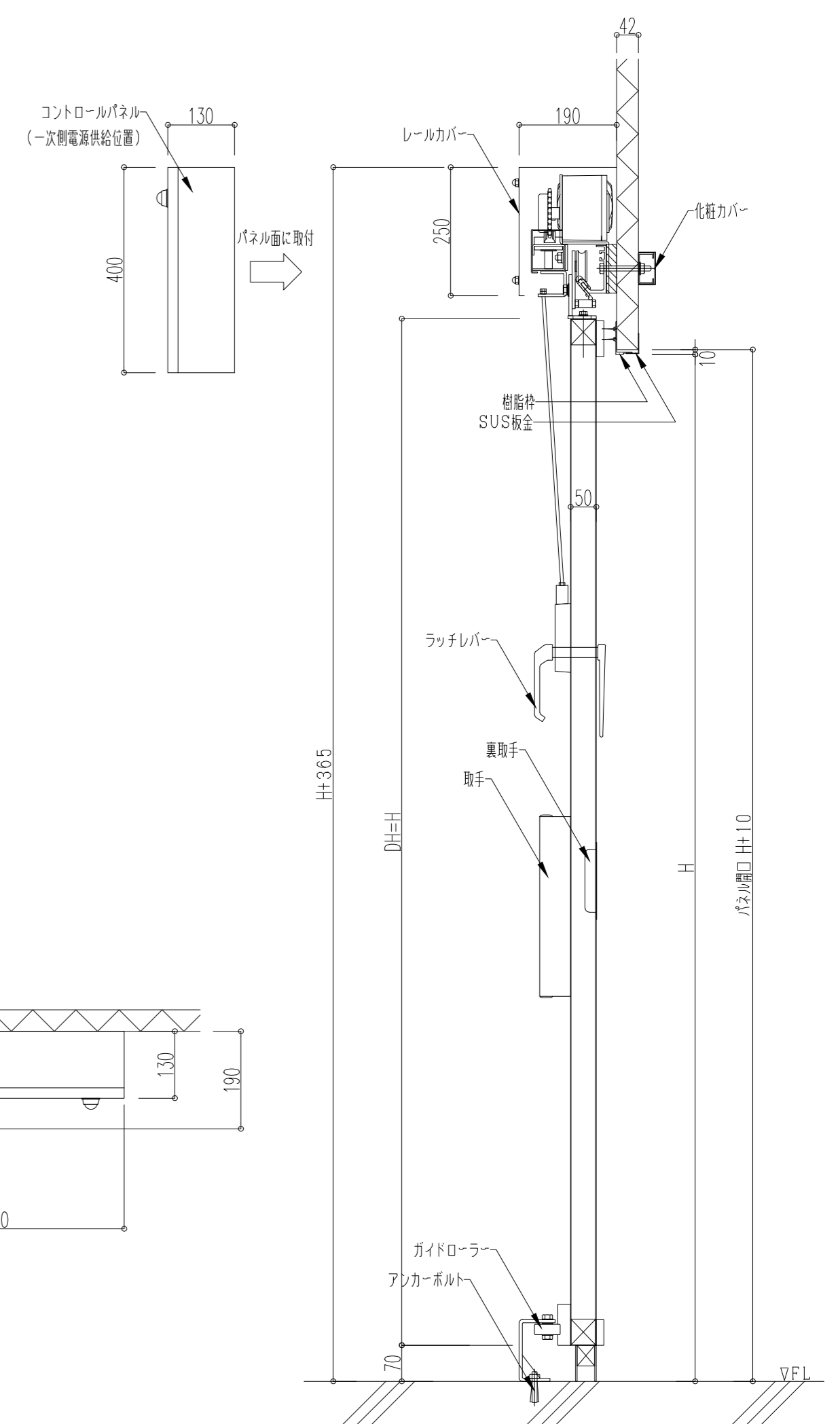
断面図 S=1/10
