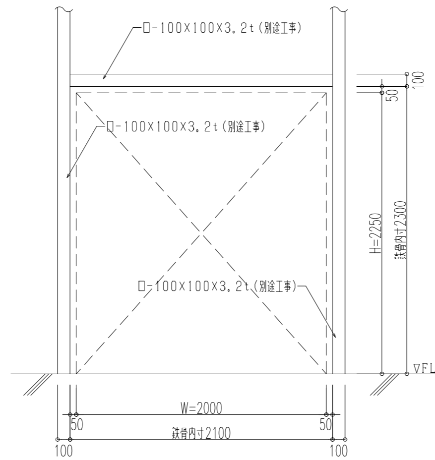
下地鉄骨寸法図 s=1/30
