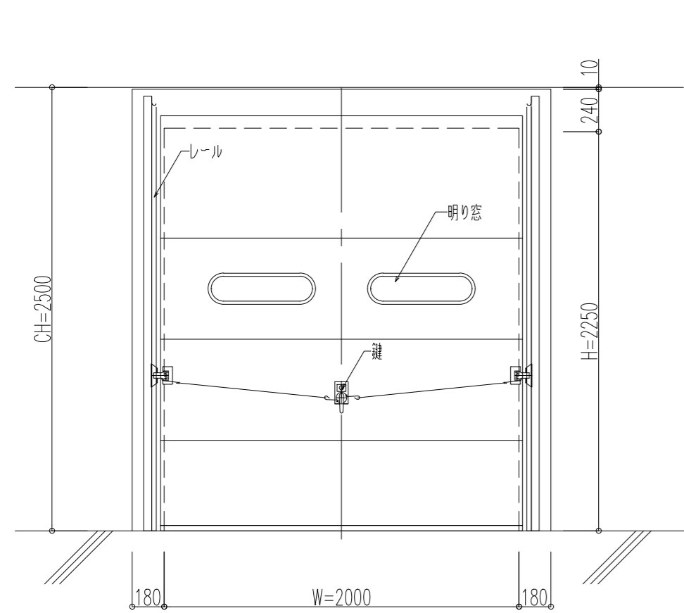
正面姿図 s=1/30
