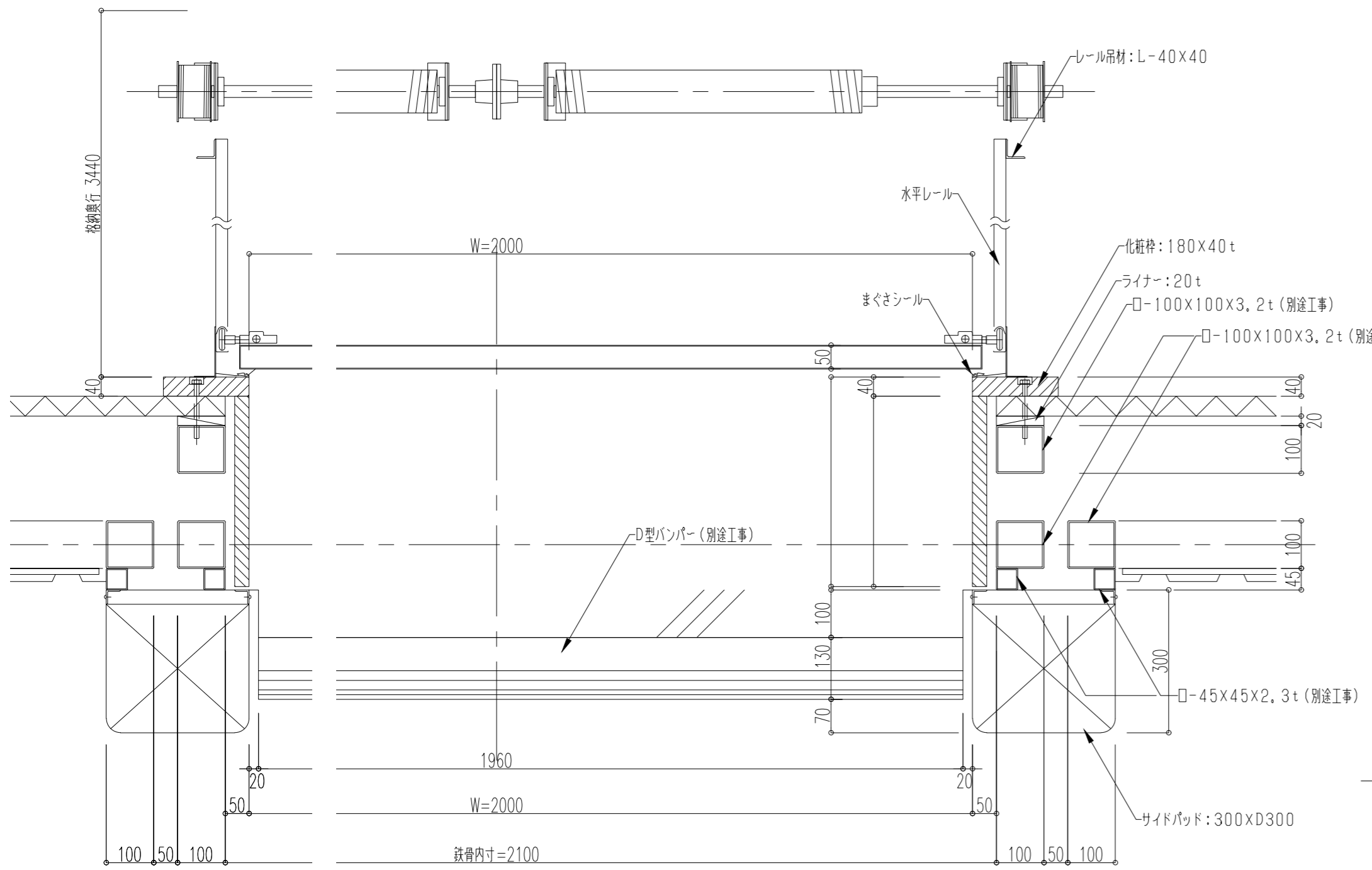
平面図 s=1/10
