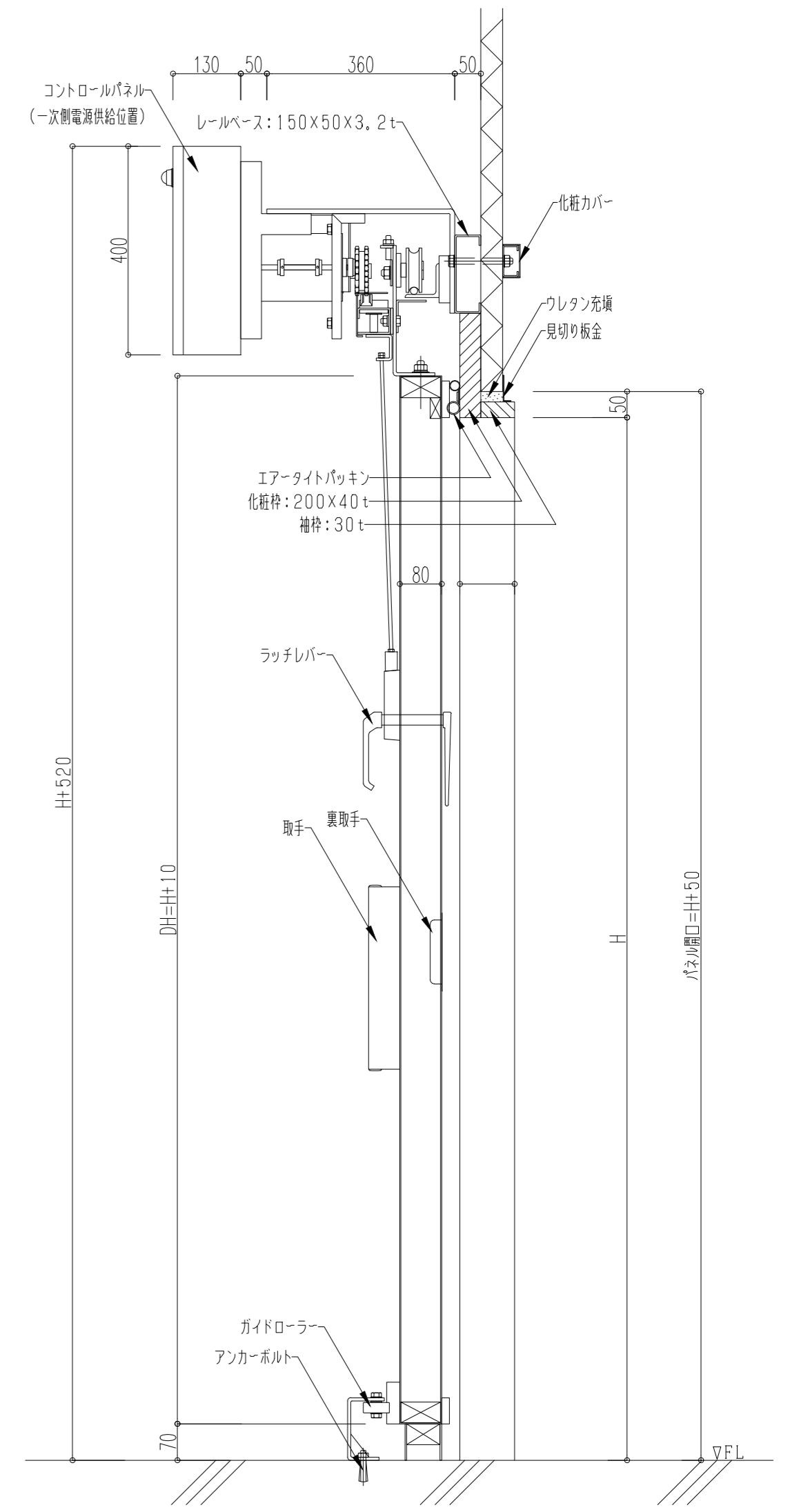
断面図 S=1/10
